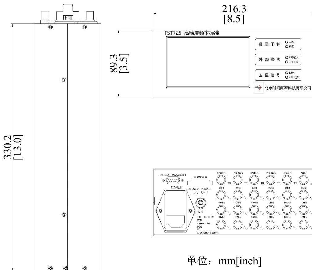
图 1FST725 结构尺寸
