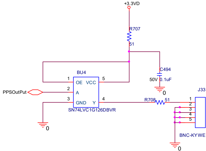
图 6PPSOUT 内部接口电路
