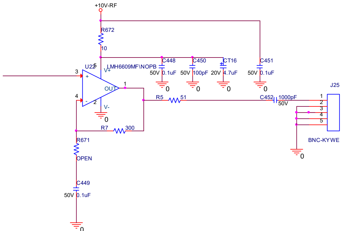
图 710MHz 接口电路
