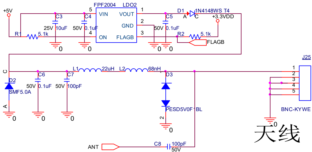
图 8GNSS 天线接口
