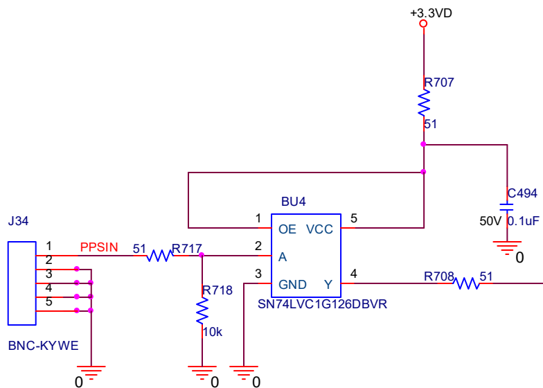
图 5PPSIN 内部接口电路
