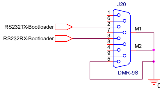
图 4RS232 接口
